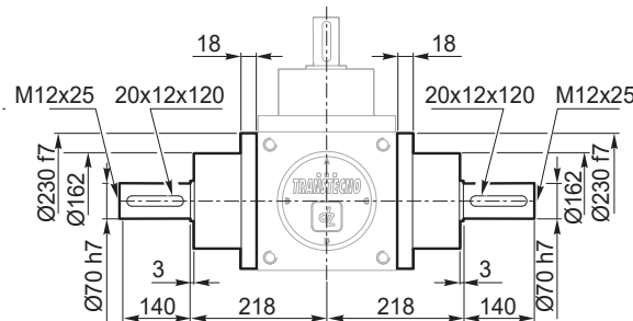
Versione rinforzata Strengthened version
