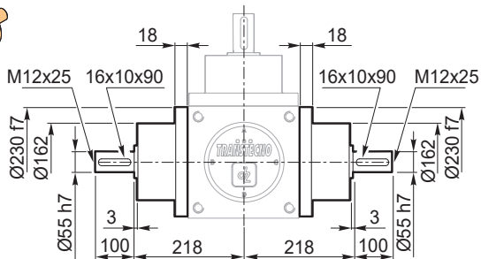
Versione standard Standard version
