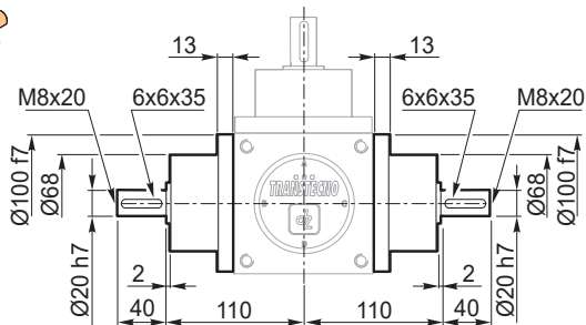
Versione standard Standard version
